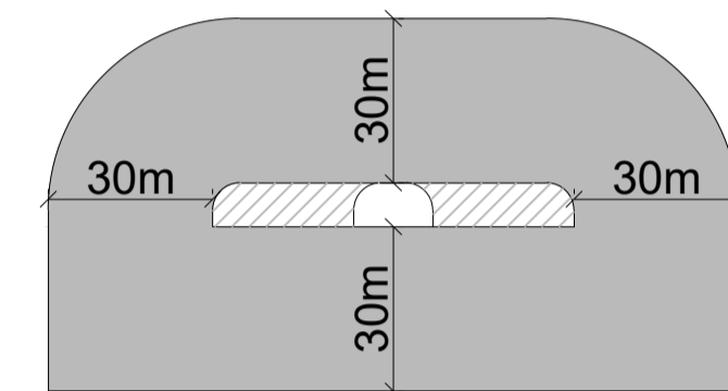
Prinsipsnitt for tunnel, hovedløp
